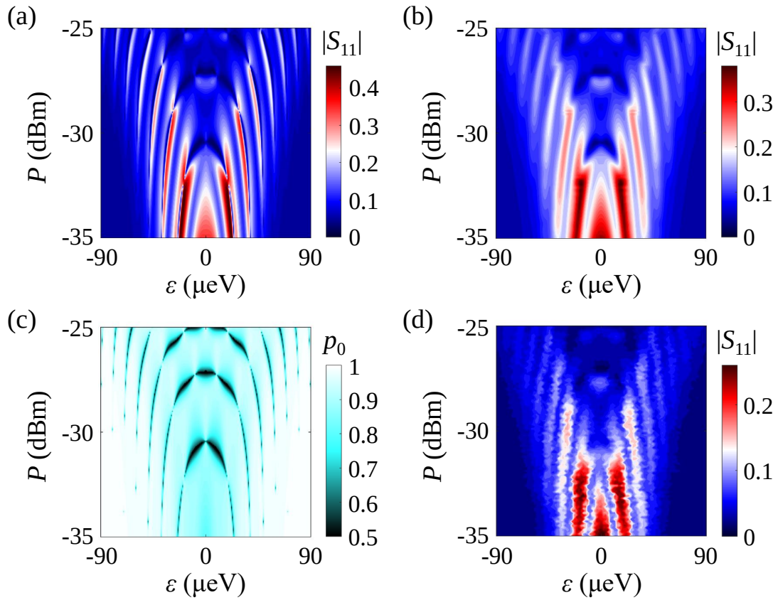
图 6.7 (a) 驱动频率 f_d = 2.27 GHz 在接近三分之一谐振频率处的理论预言结果，驱动功率 P = -29 dBm，对应幅值 A_d = 45 \mu eV。(b) 相同的数值计算，但是额外考虑了失谐量 \varepsilon 具有 2.5 \mu eV 的噪声展宽。(c) 理论计算的 Floquet 态 |\phi_0\rangle 平均布居。(d) 驱动频率 f_d = 2.27 GHz 时的谐振腔响应实验结果。
